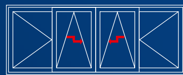
4 részes elem 2 tolószárnyal és 2 nyitható szárnyal
